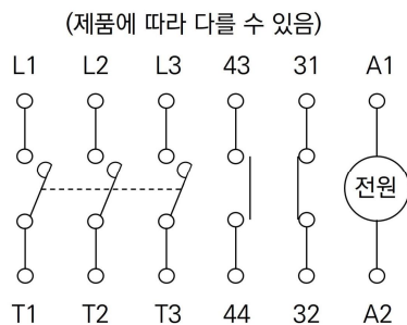
[MC 내부결선도]
